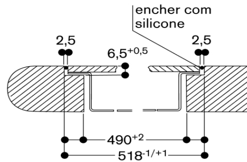
Secção transversal
