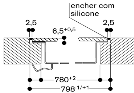
Secção longitudinal
